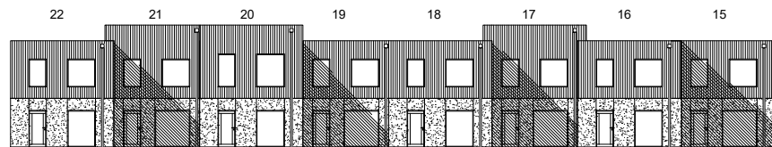
Fasad mot norr radhus 15-22
