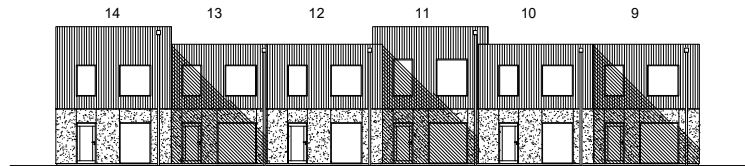
Fasad mot norr radhus 09-14
