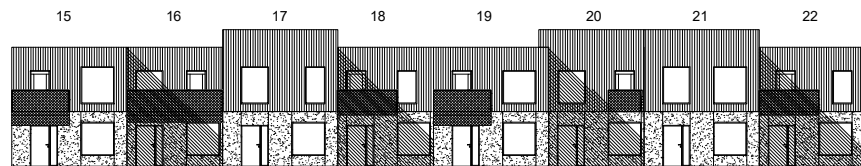
Fasad mot söder radhus 15-22
