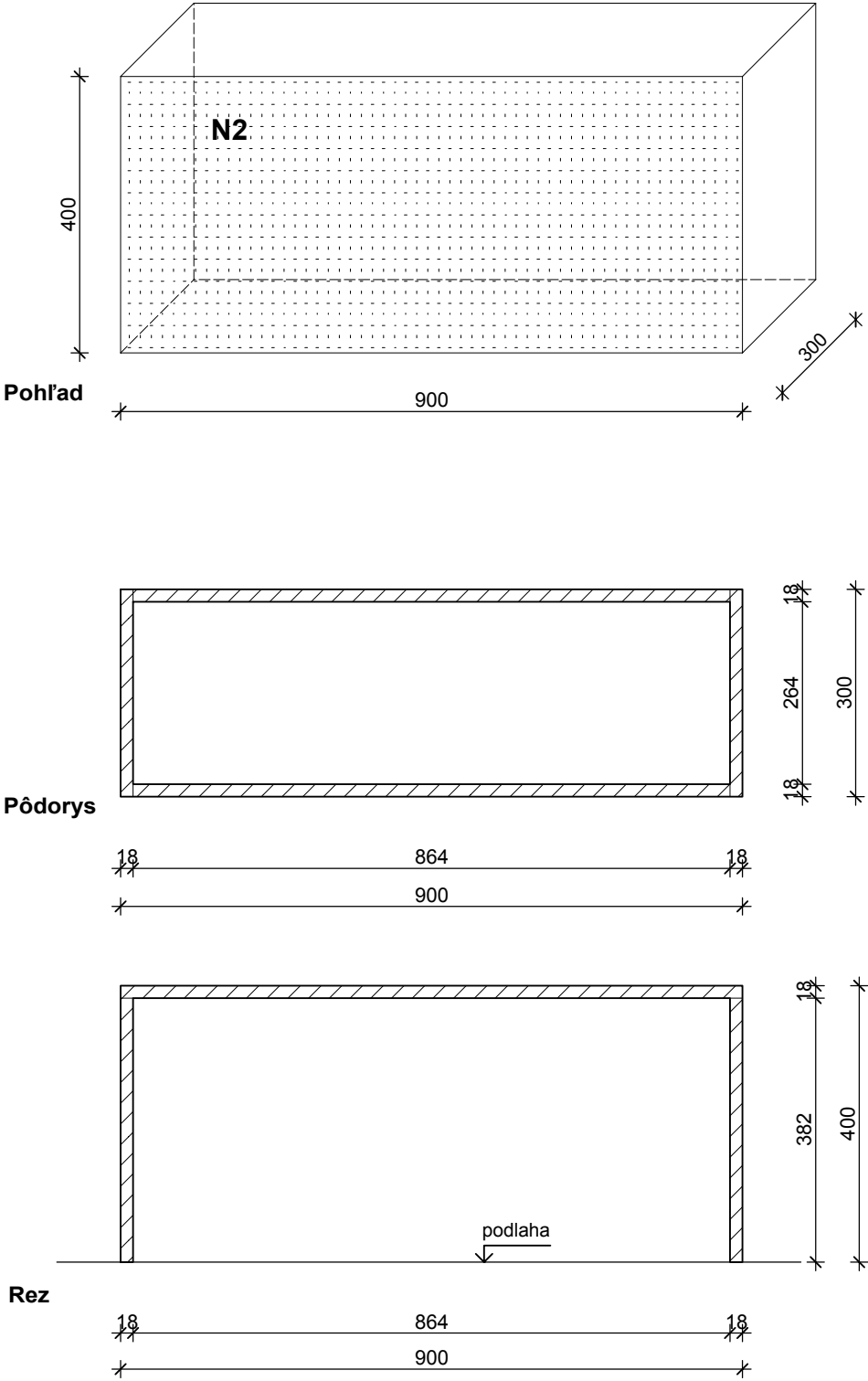
NÁBYTKOVÝ PRVOK N2
