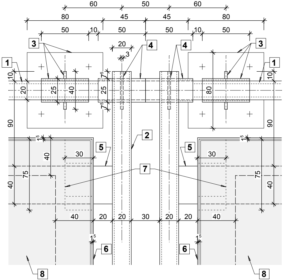
Det. "y" Pohľad na kotvenie dvoch panelov M 1 : 2,5
