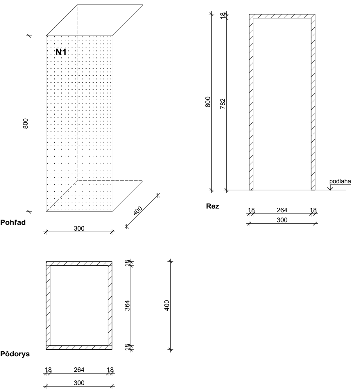
NÁBYTKOVÝ PRVOK N1
